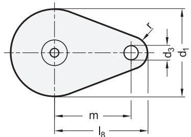
Pohled shora
