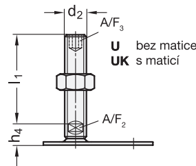
Provedení se závitovým čepem
