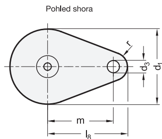
Pohled shora
