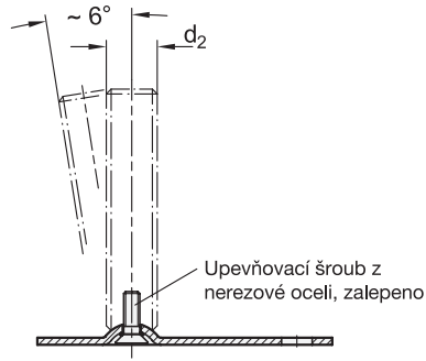
Provedení se závitovým čepem
